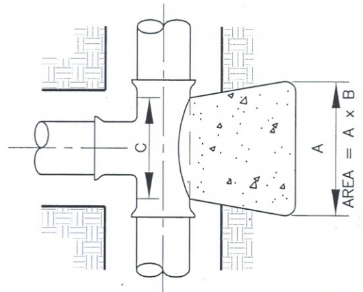
TEE
